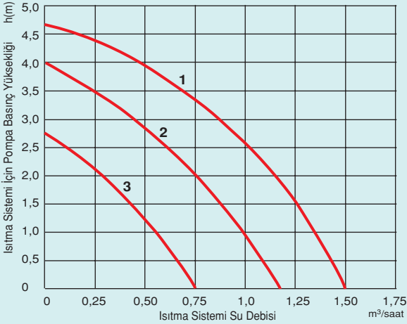
Sirkülayon Pompası Performans Grafiği
